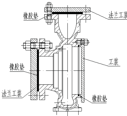
图4 改进后的试压方法（泵体零件）
