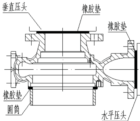
图3 传统试压方法（泵体零件）
